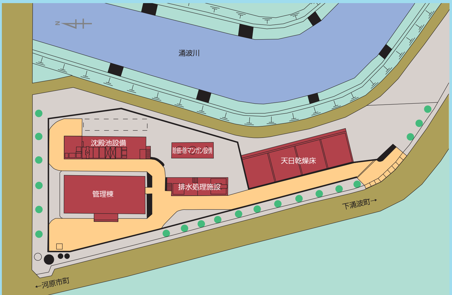
▼金沢市工業用水道 金沢テクノパーク浄水場平面図
